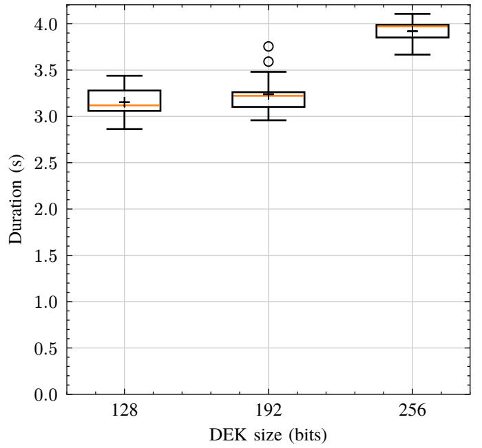
Fig. 5b. KeyUnwrap box-plot distribution per parameter set (tiny corpus only; linear y axis)
